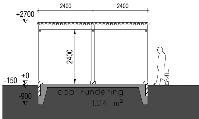
doorsnede schuur
