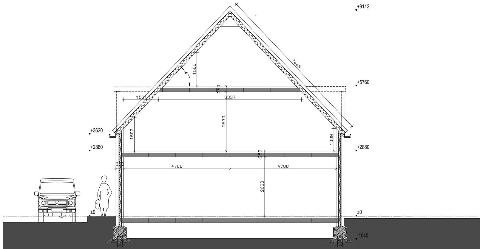
doorsnede B - B woningen 3 t/m 10
